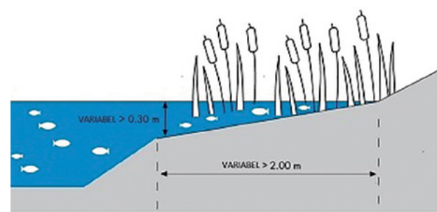
Natuurvriendelijke oever
