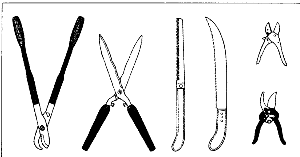
Snoeigereedschap. Van links naar rechts: snoeischaar met lange handvatten, speciaal voor dikke takken; heggeschaar; boomzagen voor grote takken; rechte en gebogen snoeischaar voor het snoeien van heesters.
